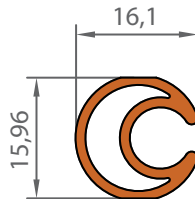
1009 0,231 KG/M
