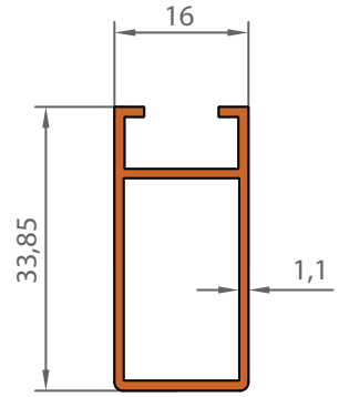
1010 0,307 KG/M
