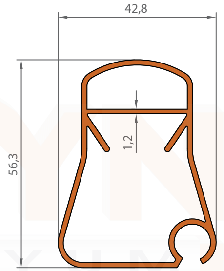
1002 0,865 KG/M
