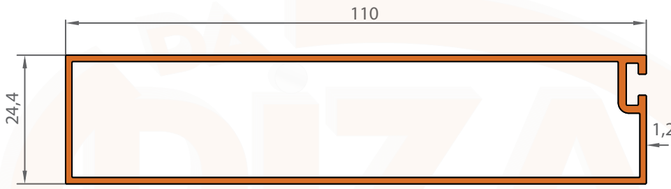
1133 0,897 KG/M
