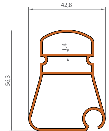
1001 0,916 KG/M
