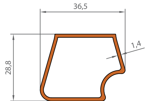
1003 0,426 KG/M
