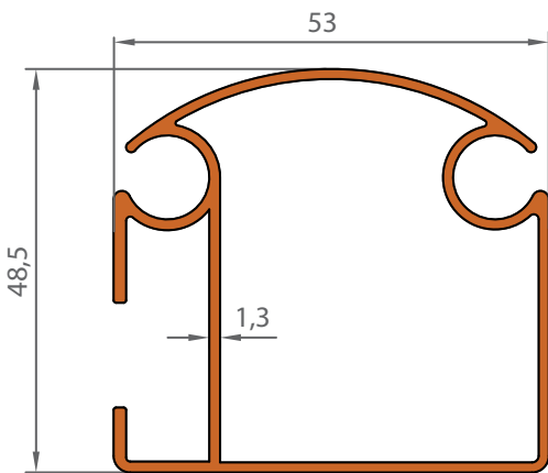
1008 0,813 KG/M
