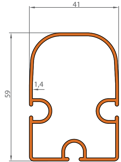
1137 0,886 KG/M
