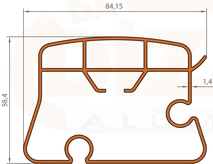
1004 1,635 KG/M
