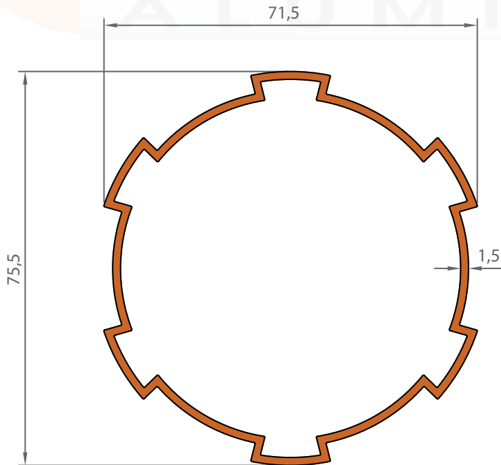
1007 1,076 KG/M
