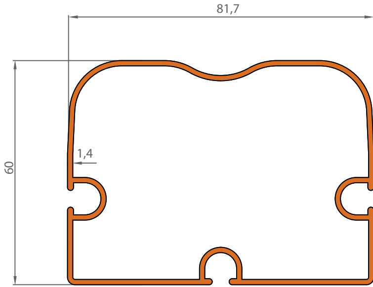
1136 1,211 KG/M
