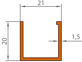
1051 0,242 KG/M
