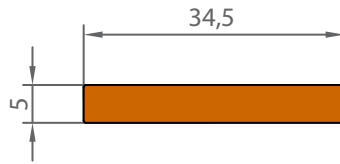
1052 0,472 KG/M
