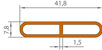
ÇITA KALIBI 0,334 KG/M
