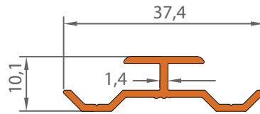
1269 0,201 KG/M
