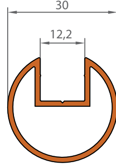
1066 0,429 KG/M
