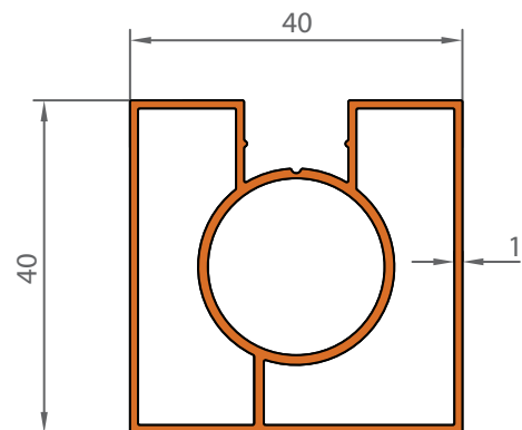
1207 0,656 KG/M
