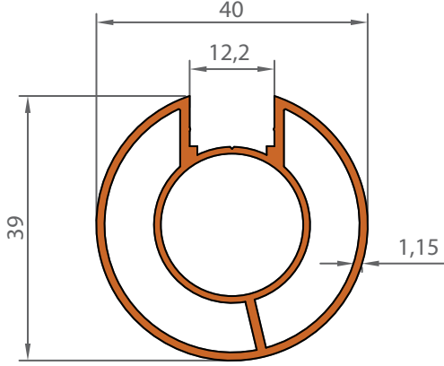
1065 0,645 KG/M
