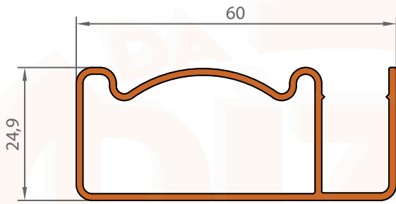
1073 0,621 KG/M
