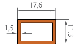
1079 0,211 KG/M
