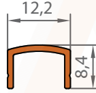
1069 0,079 KG/M
