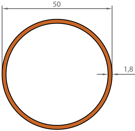
1067 0,740 KG/M
