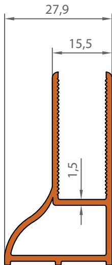
1075 0,594 KG/M
