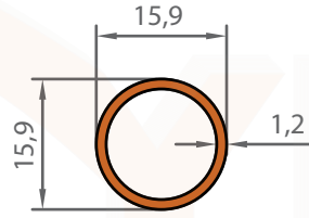
1068 0,152 KG/M
