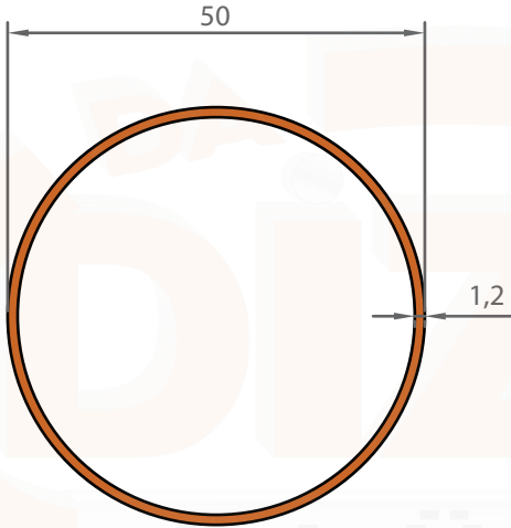
1095 0,499 KG/M
