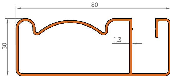
1234 0,867 KG/M
