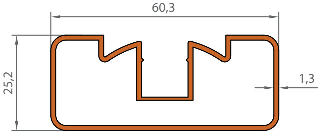
1071 0,694 KG/M
