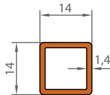
1078 0,190 KG/M
