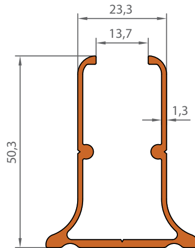
1076 0,656 KG/M
