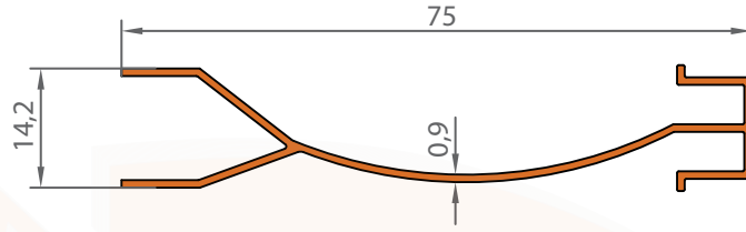
1222 0,317 KG/M
