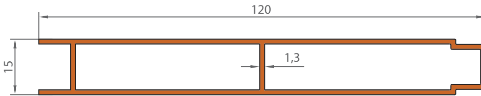
1169 0,108 KG/M
