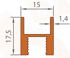
1173 0,249 KG/M
