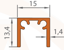
1170 0,160 KG/M
