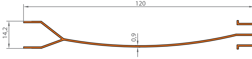
1221 0,428 KG/M
