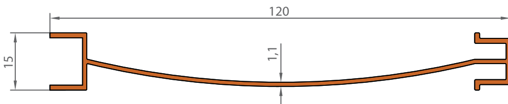
1194 0,536 KG/M
