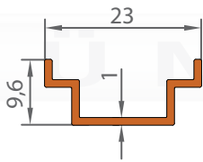
1169 0,108 KG/M
