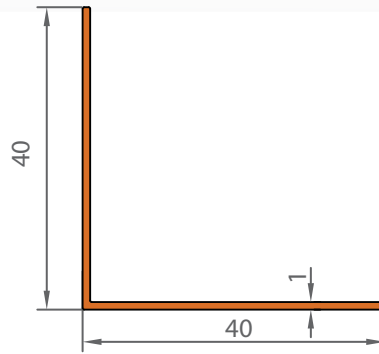
I217 0,214 KG/M
