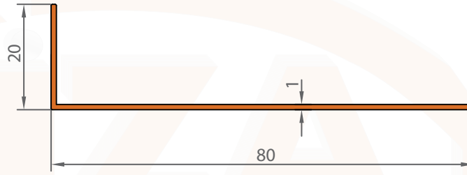
I219 0,268 KG/M
