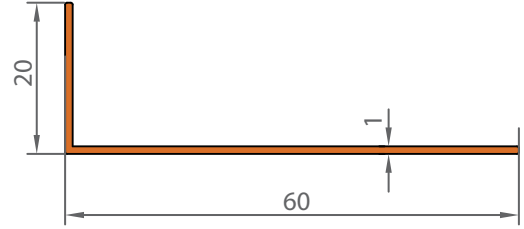
I218 0,214 KG/M
