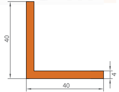
I244 0,825 KG/M
