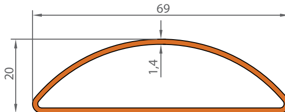
1239 0,564 KG/M
