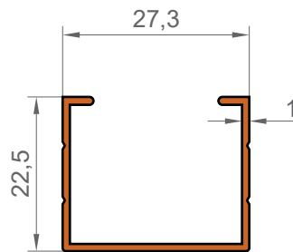
1261 0,217 KG/M
