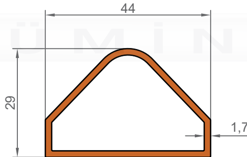
1289 0,540 KG/M
