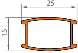
1262 0,206 KG/M
