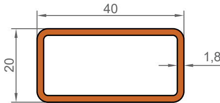
1420 0,531 KG/M
