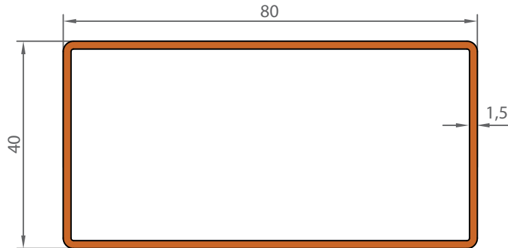
4004 0,944 KG/M
