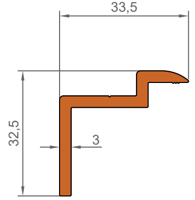
7003 0,496 KG/M
