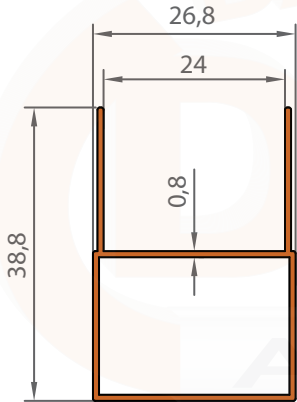
1080 0,280 KG/M
