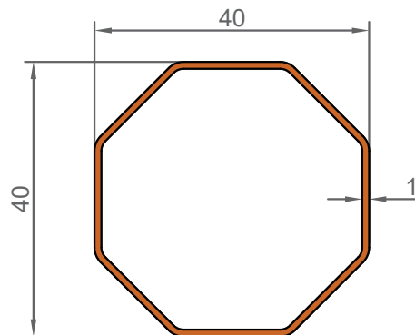
1384 0,347 KG/M
