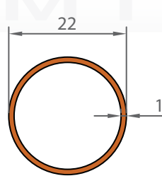
1109 0,178 KG/M
