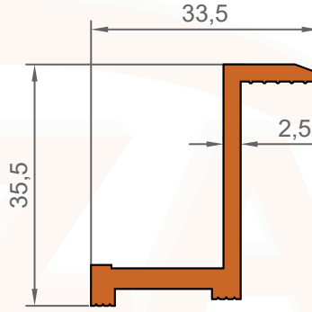
1446 0,501 KG/M
