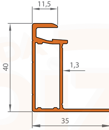
6004 0,491 KG/M
