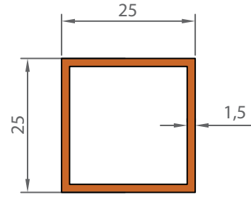
1114 0,385 KG/M
