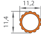
1156 0,081 KG/M
