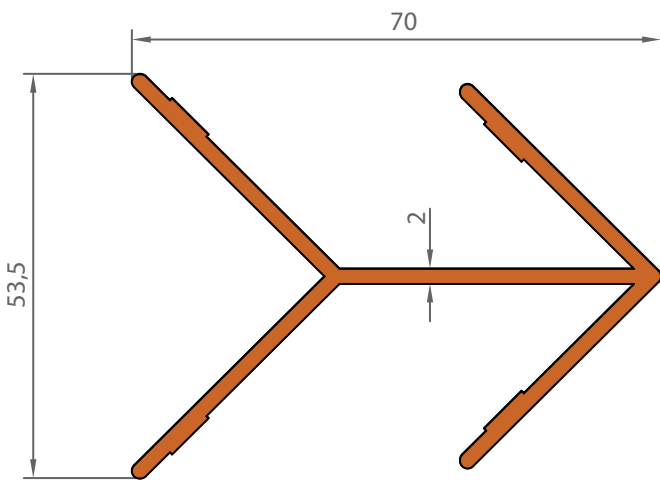
1064 1,071 KG/M
