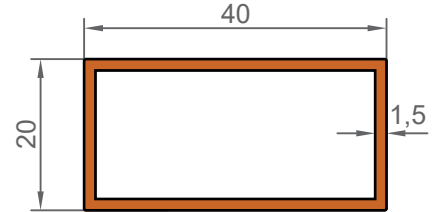
1241 0,463 KG/M
