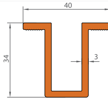
1119 0,826 KG/M
