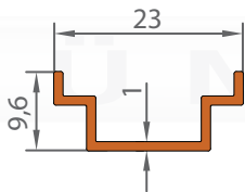
1169 0,108 KG/M
