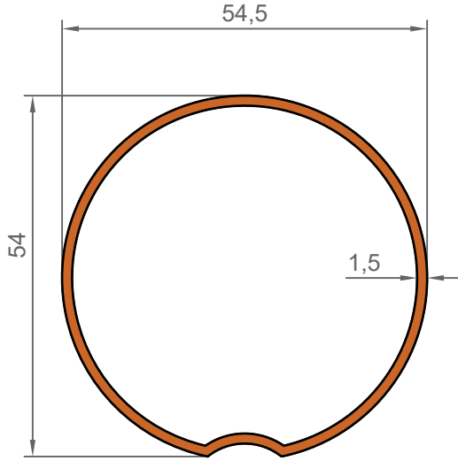
1280 0,678 KG/M
