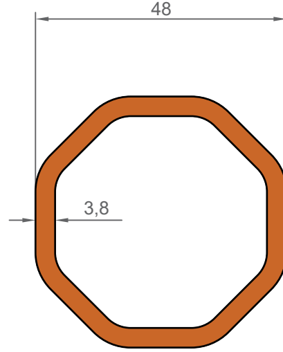
1273 1,463 KG/M
