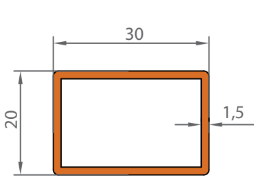
1242 0,379 KG/M
