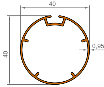
1026 0,391 KG/M
