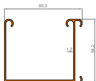
1148 0,623 KG/M
