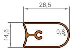
1021 0,204 KG/M
