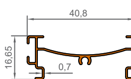
1038 0,198 KG/M
