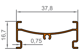
1037 0,187 KG/M
