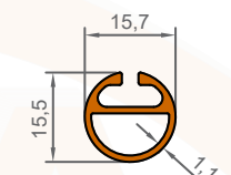
1039 0,187 KG/M
