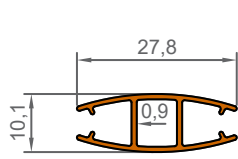
1029 0,177 KG/M
