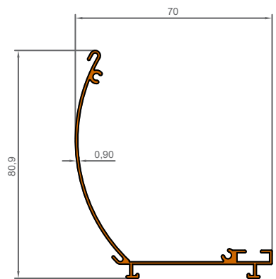
1032 0,494 KG/M
