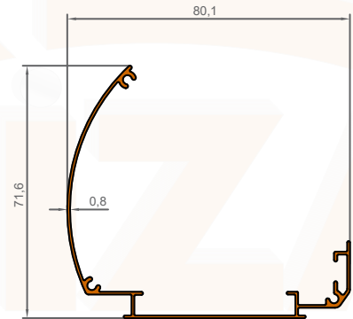
1019 0,467 KG/M
