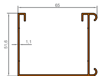
4012 0,605 KG/M
