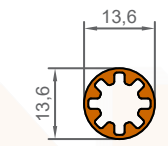
1022 0,174 KG/M
