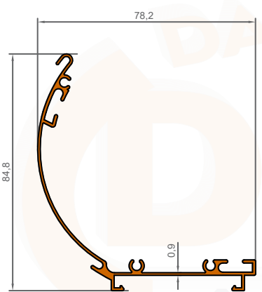
1045 0,637 KG/M
