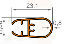
1027 0,163 KG/M
