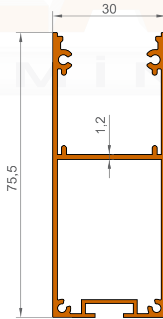
1111 0,832 KG/M
