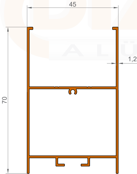
1102 0,916 KG/M
