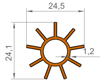
1017 0,282 KG/M
